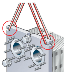
Figure 5 : Levage des modèles AQ1, AQ2, AQ4, AQ1A, AQ2A, AQ2S, AQ1L et de l'ancienne version du modèle AQ3, AQ2L
