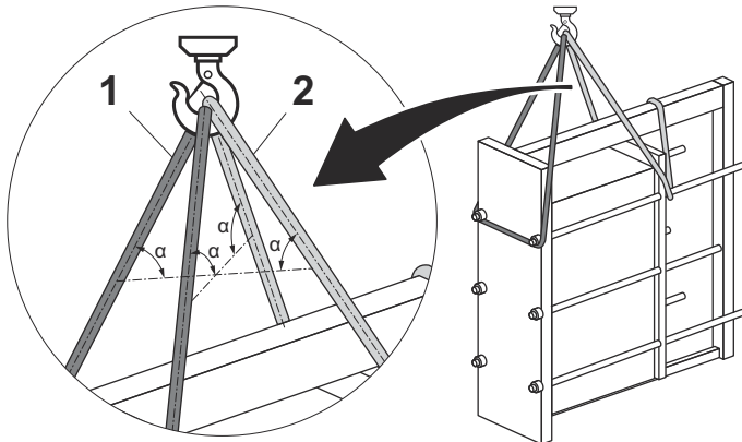
Figure 4 : L'illustration montre le filetage des élingues.
