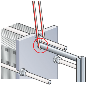
Figure 6 : Levage des modèles AQ1, AQ2, AQ4, AQ1A, AQ2A, AQ1L et de l'ancienne version du modèle AQ3, AQ2L
